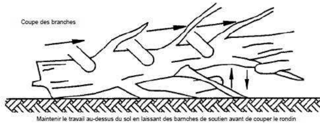
Figure BB.103 – Ébranchage d'arbre
